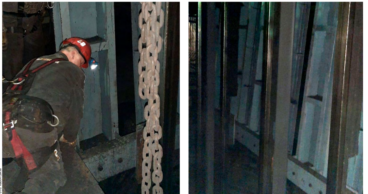
Výměna lan na skipovém těžním zařízení č. 4 na severní lokalitě stonavské šachty.
